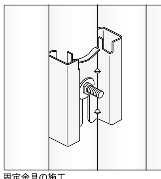
固定金具の施工
