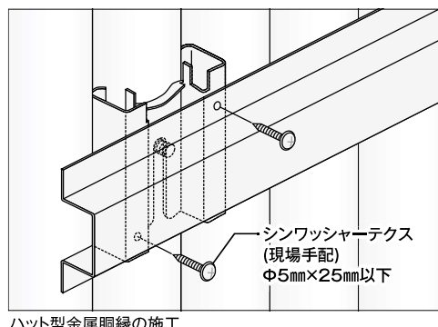
ハット型金属胴縁の施工
