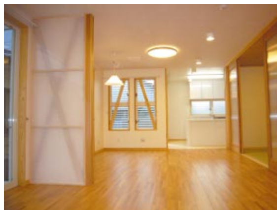
住宅の筋かい
